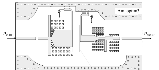
Fig.2 Layout of the circuit 图 2 电路版图
