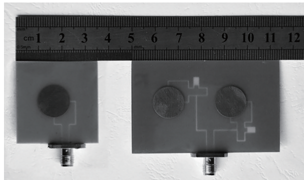
Fig.9 Views of antenna and array 图 9 天线及线阵加工实物图
