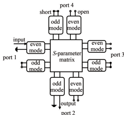
Fig.2 Schematic diagram of the converter 图 2 共面波导-槽线转换器原理图
