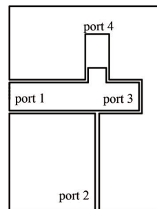
Fig.3 Layout of the converter 图 3 转换器版图
