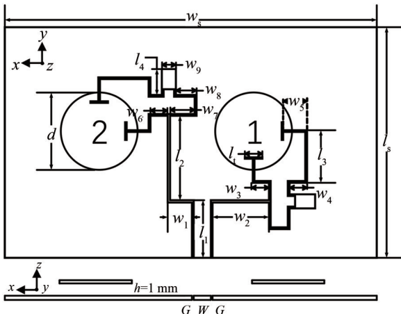
Fig.8 Geometry of the 1\times 2 array 图 8 1\times 2 阵列天线结构示意图
