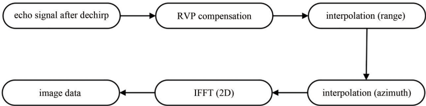
Fig.6 Polar format algorithm 图 6 极坐标格式算法
